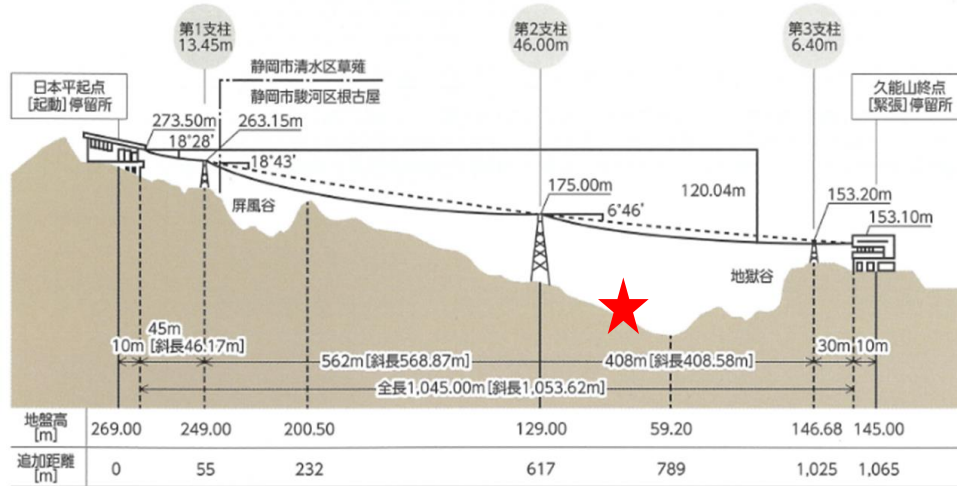
線路縦断面図
